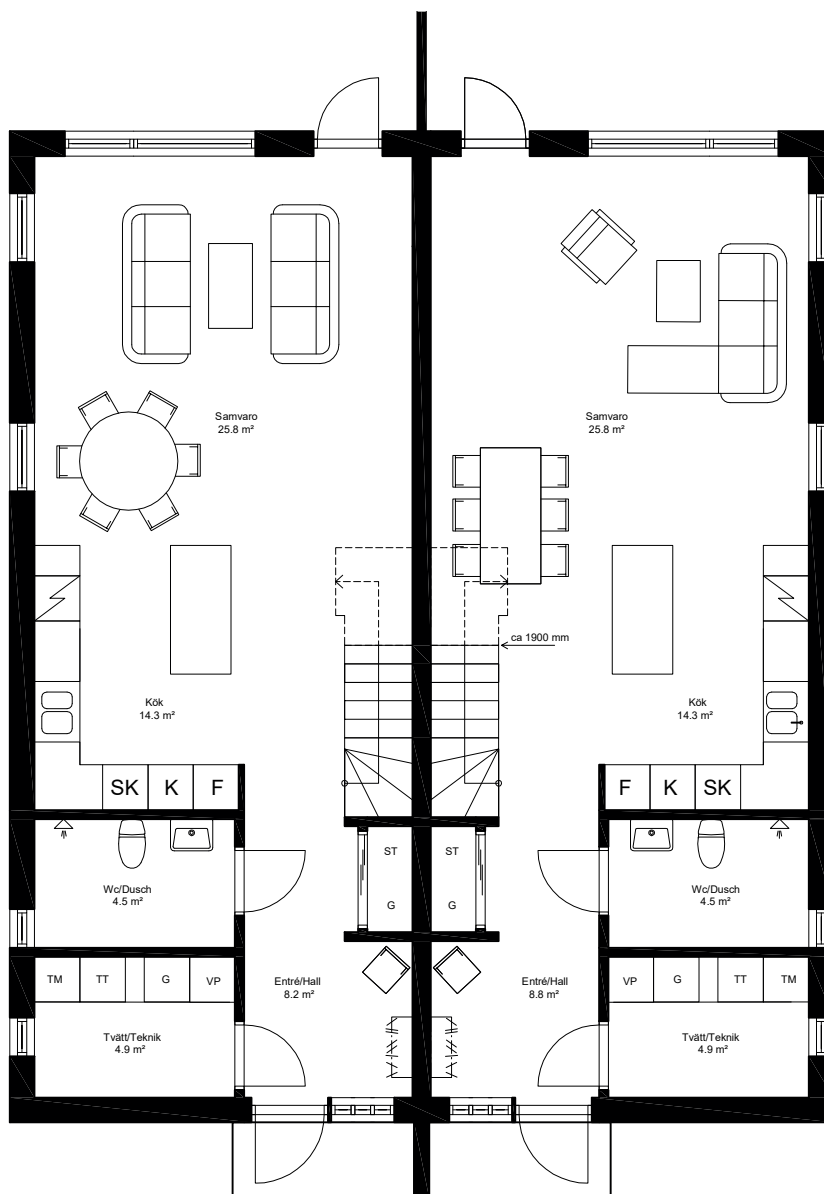
Entréplan
